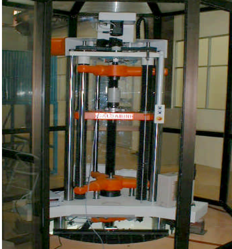
Patrón Nacional de Fuerza de 50 kN hasta 150 kN.
